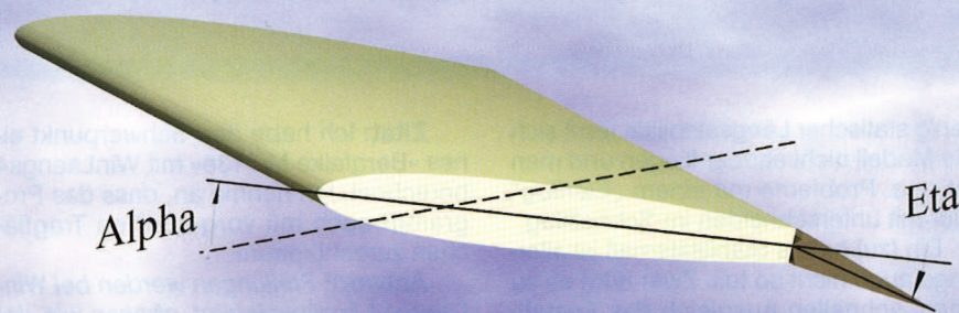
Definition von Flossenstellwinkel Alpha und Höhenruderklappenwinkel Eta
